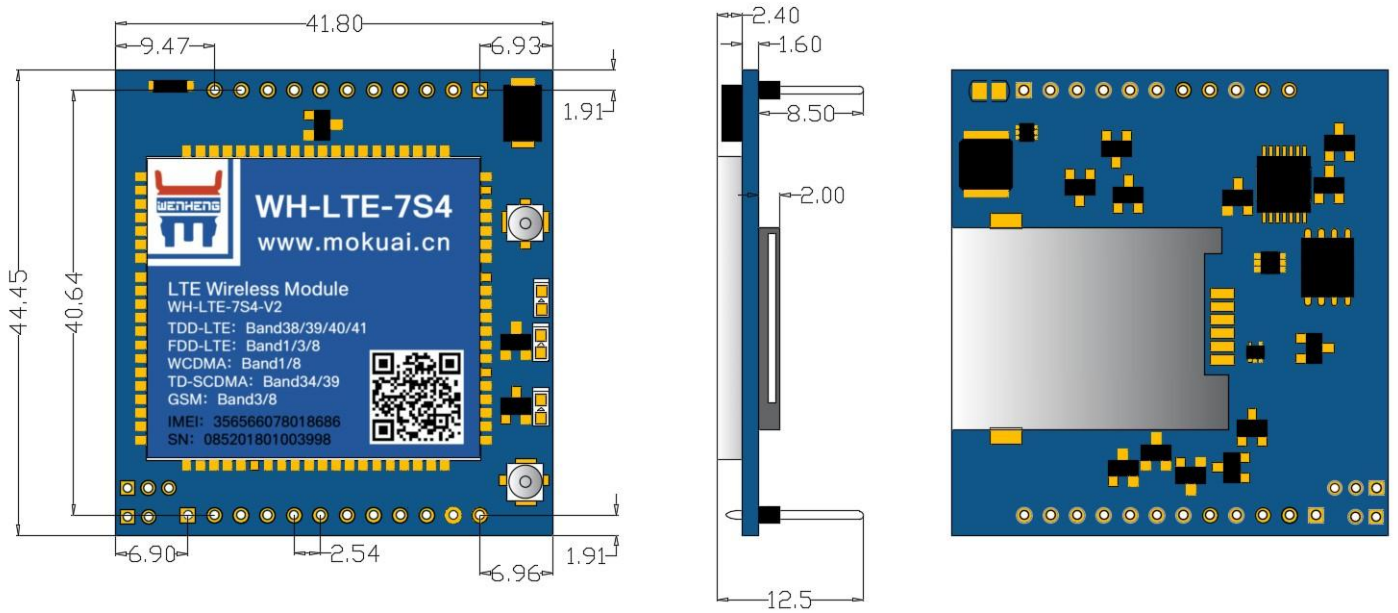
图 3 模块尺寸图
