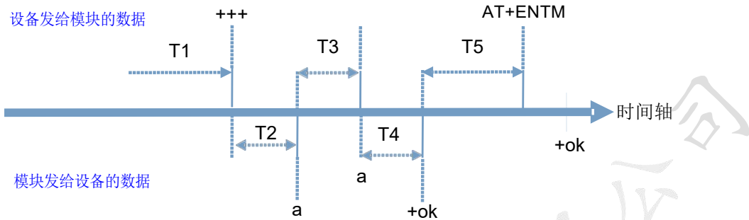
图 20 切换指令模式时序
